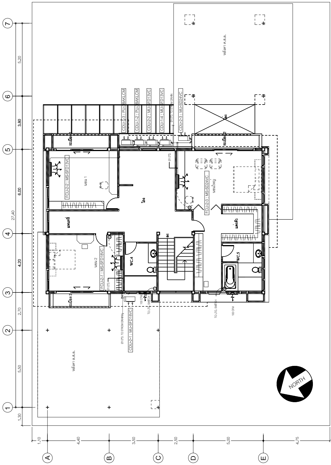
แปลนพื้นที่ห้อง ขนาดกระดาษ 1:100
